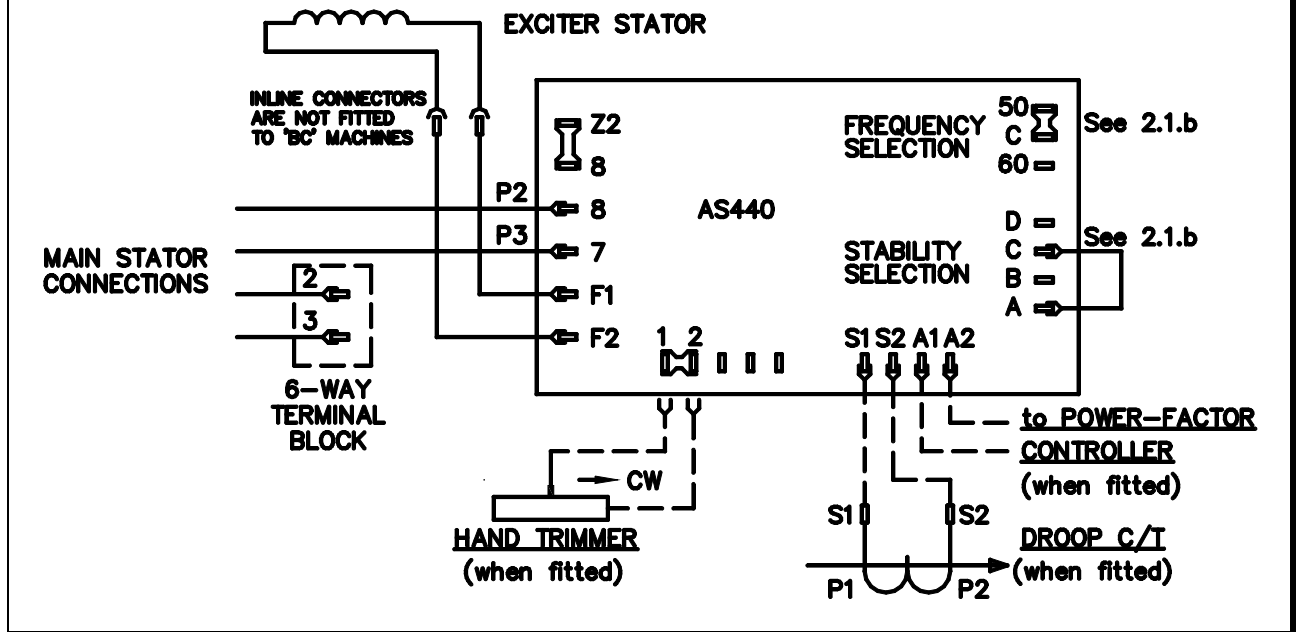
Fig 4 : New wiring for the AS440 AVR.
